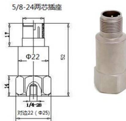
外形尺寸
